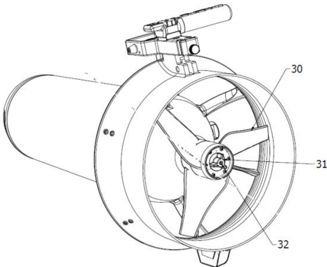
Fig.9 - Estrazione dell'elica
