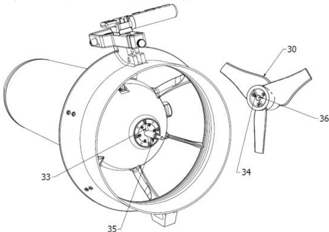
Fig.10 - Inserimento dell'elica
