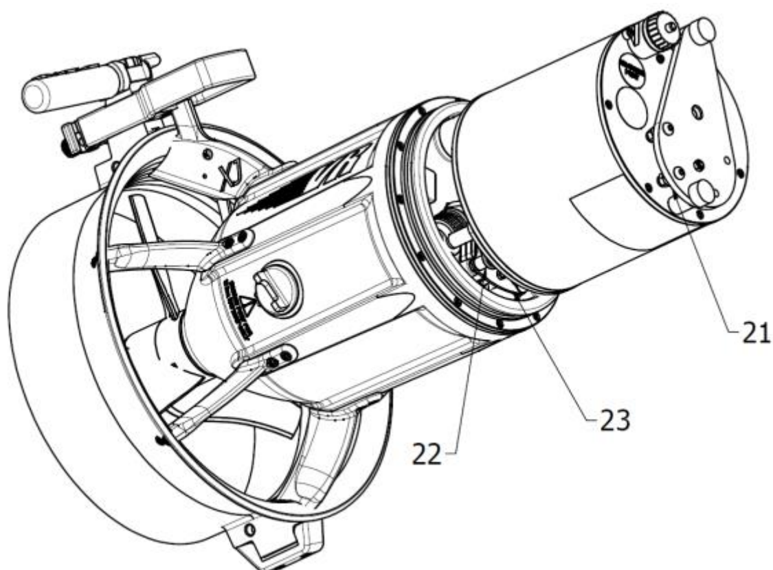
Fig.7 - Inserimento della zavorra
