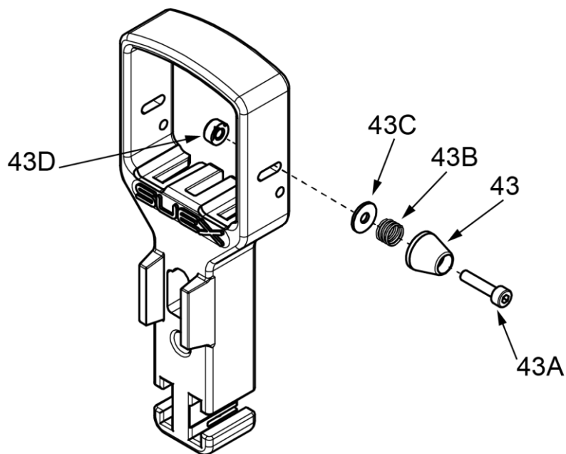
Fig 21 - Posizionare il Cruise control sul lato destro
