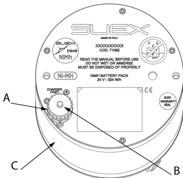
Fig 25 - VRT - batteria NiMh
