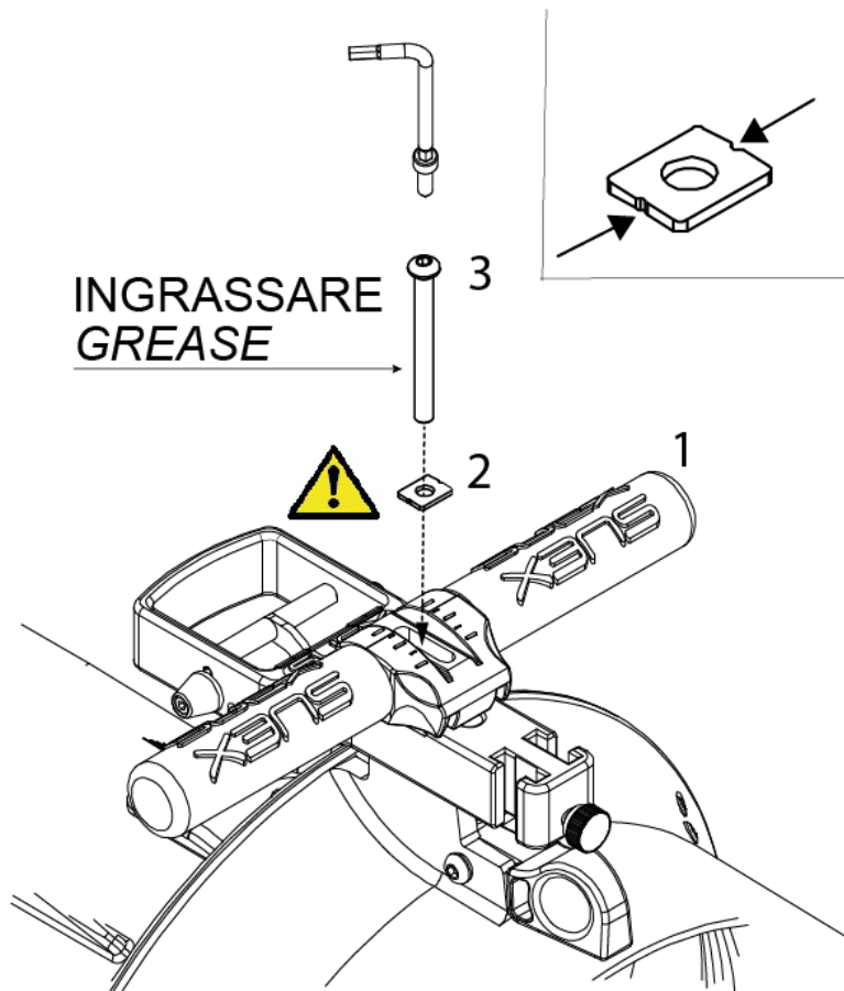
Fig 6 - Installazione impugnatura
