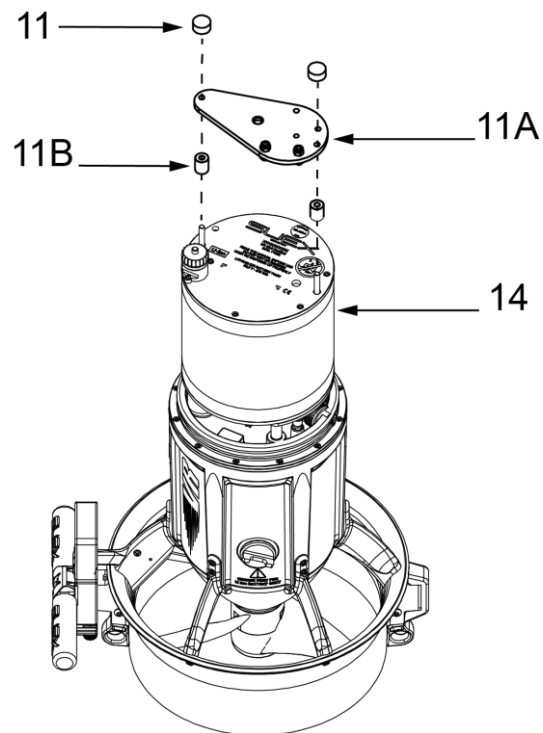
Fig 29 - Inserimento batteria
