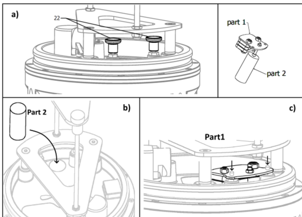
Fig 15 – Ballast insert
