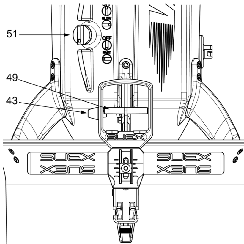
Fig 16 - Comandi dello Scooter
