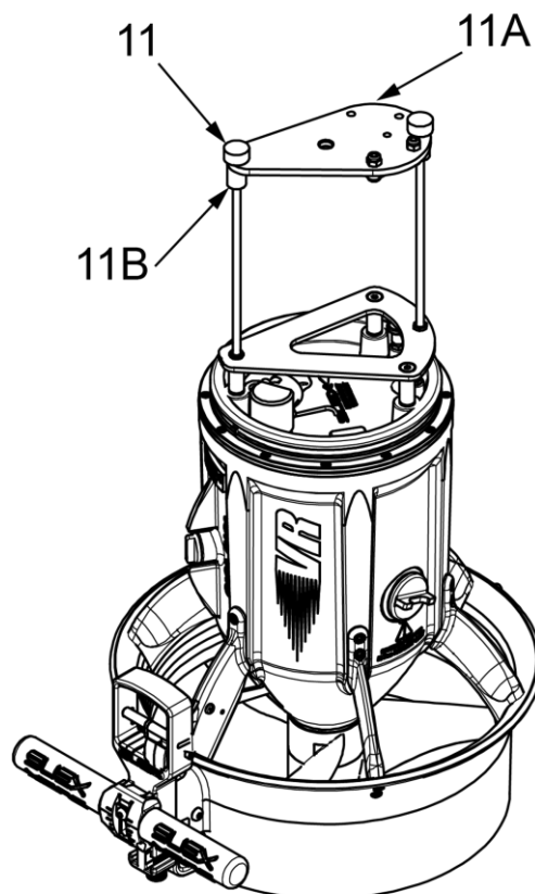
Fig 27 - Rimozione della piastra
