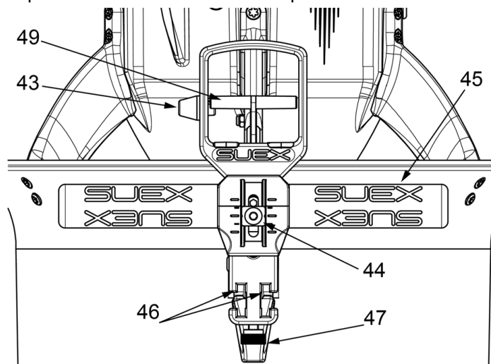
Fig 17 - Comandi sull'impugnatura
