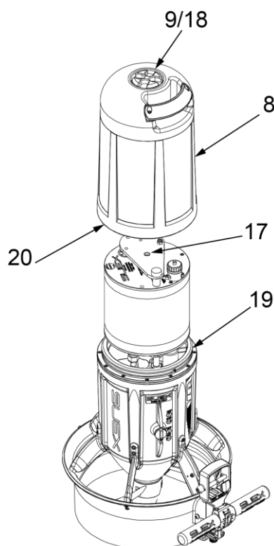
Fig 30 - Chiusura del vano batteria
