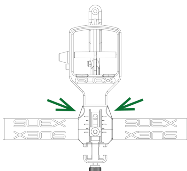
Fig 8 - Installazione impugnatura contraria
