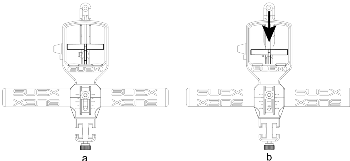
Fig 18 - Posizione grilletto
