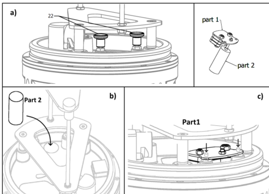
Fig 15 - Inserimento zavorra
