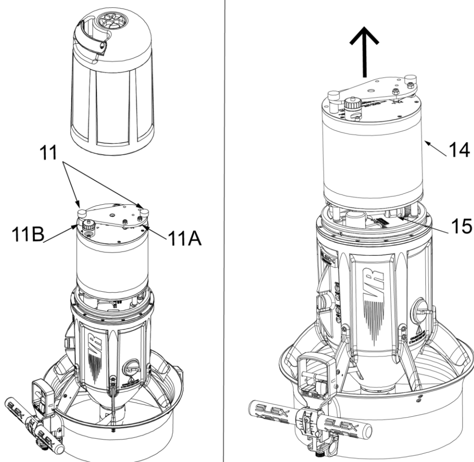
Fig 24 - Apertura vano batteria
